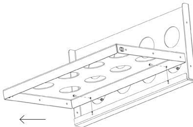
M8X16 | M8 Zinc | Dome nut M8 x4
